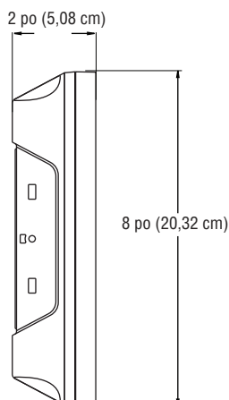
VUE LATÉRALE
