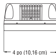
VUE DU
