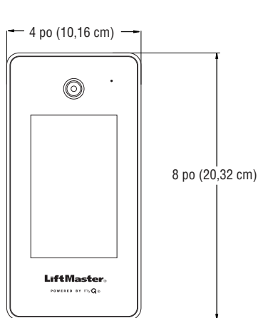
VUE AVANT
